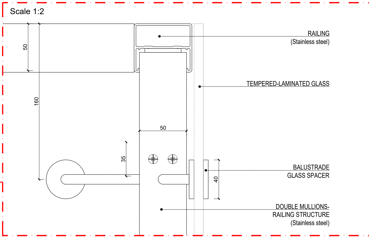
Scale 1:2
