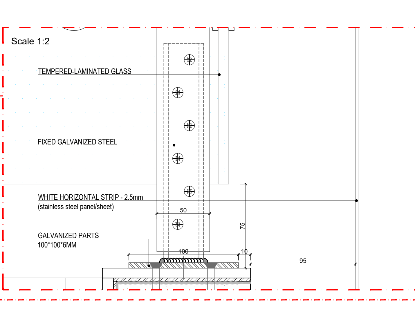
1b Section AA SCALE: 1:2
