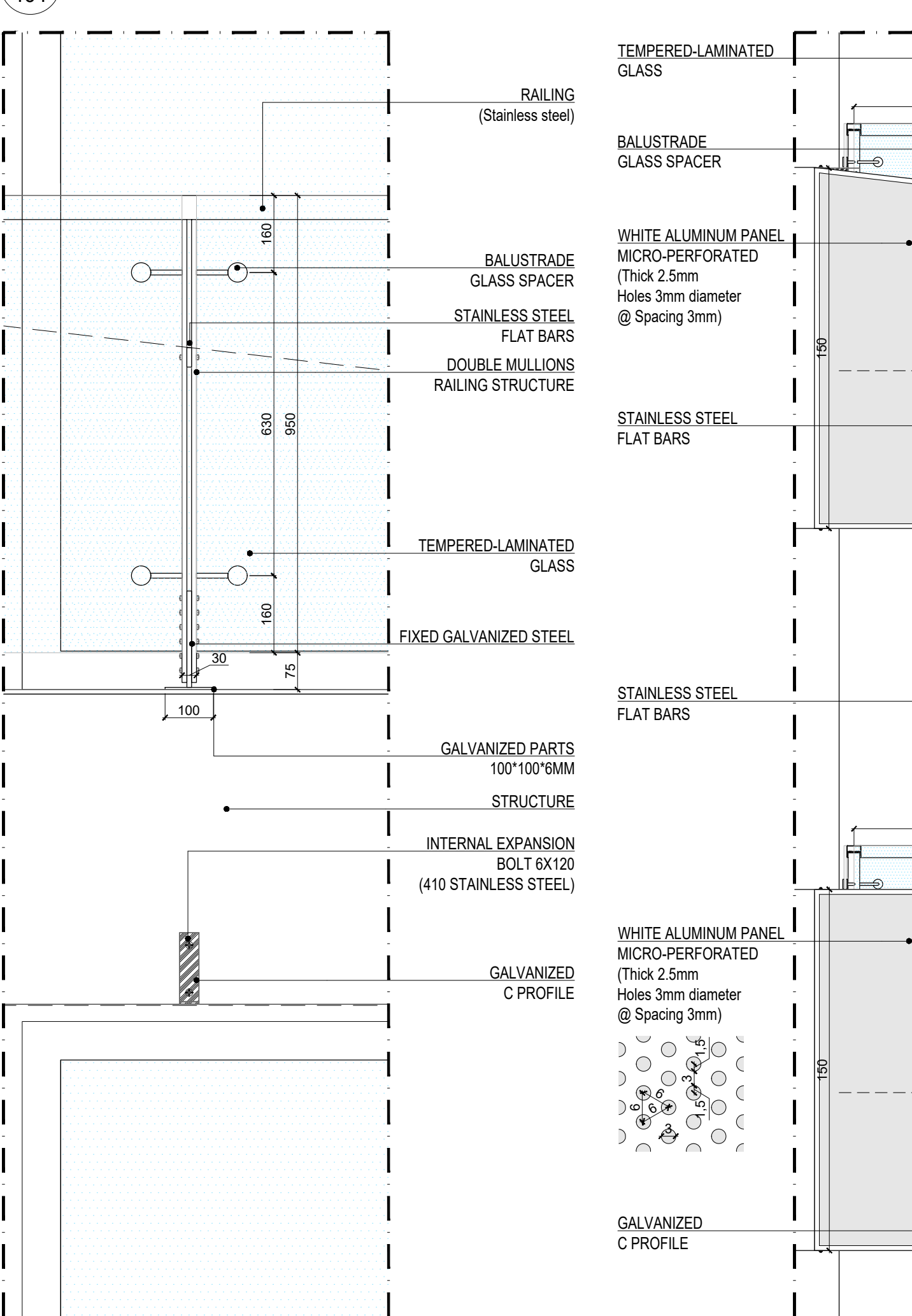
2 Section BB SCALE: 1:10
