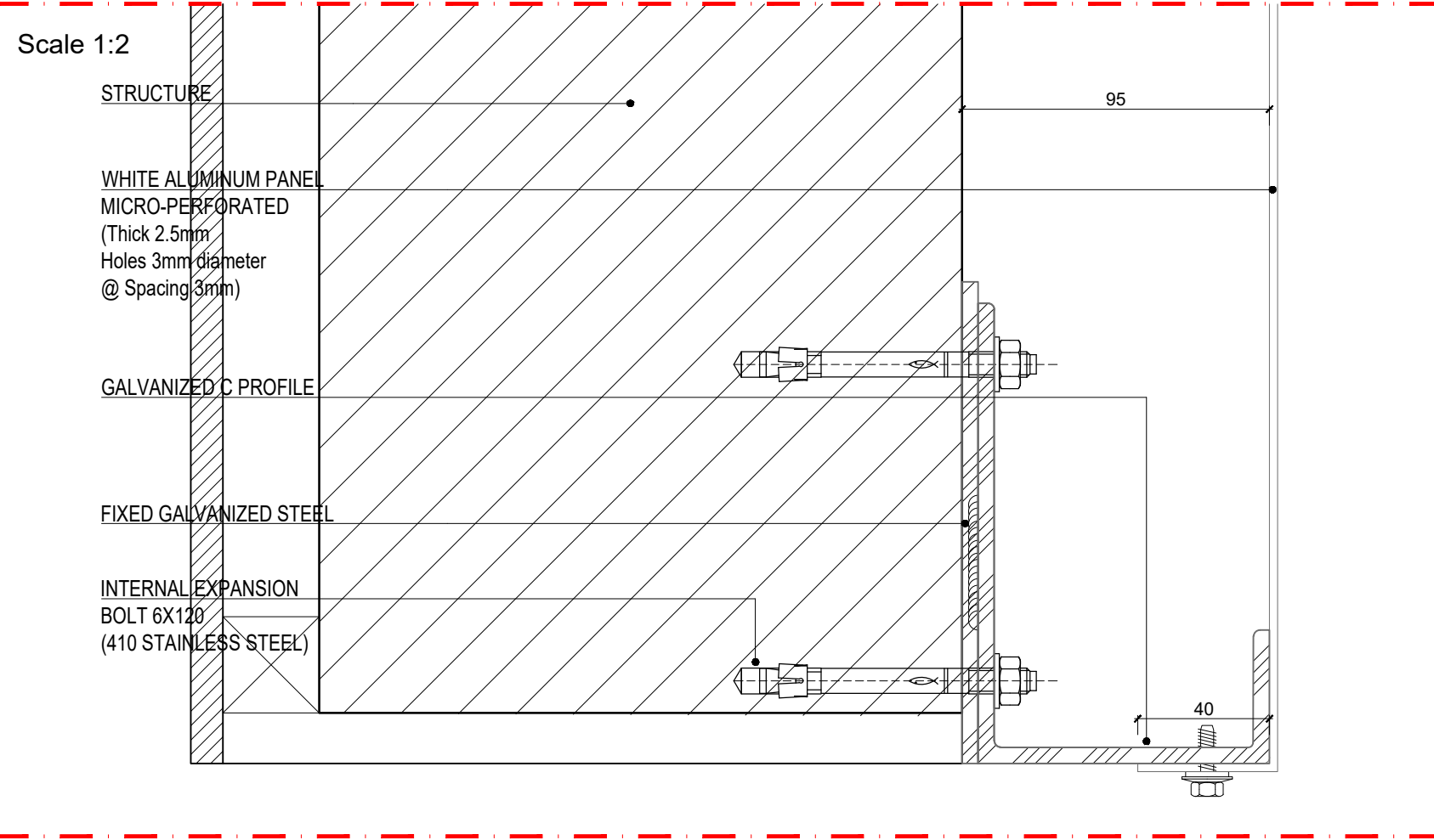
Scale 1:2
