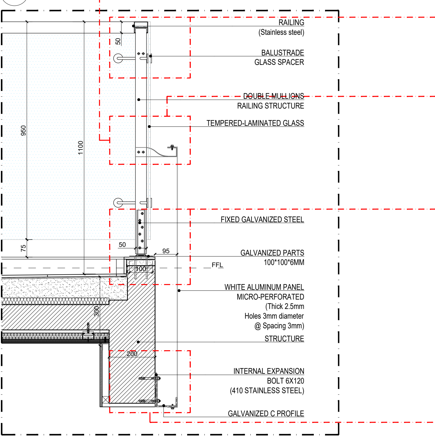
1a Section AA SCALE: 1:10
